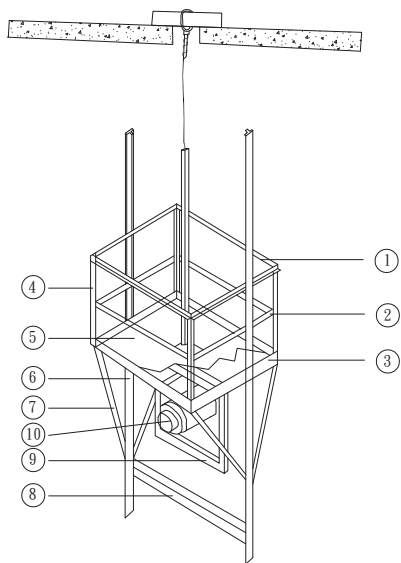
無架電梯施工平台
