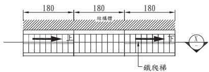
鐵爬梯平面圖
