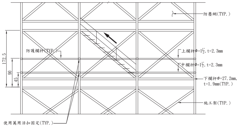
欄杆扶手細部圖
